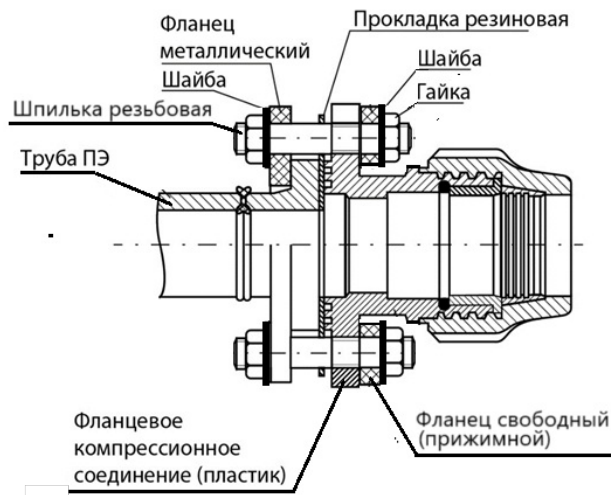
Рисунок 17 - Фланцевое компрессионное соединение в сборе
