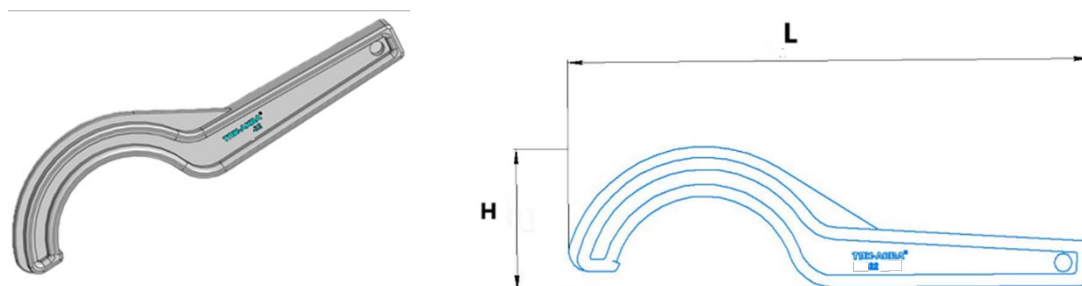
Рисунок 18- Ключ для гаек компрессионных фитингов dn 32 ТПК-АКВА
