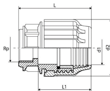
Рисунок 4 - Муфта с внутренней резьбой
