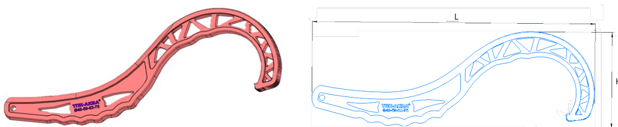
Рисунок 19. Ключ для гаек компрессионных фитингов dn 40-50-63-75 ТПК-АКВА
