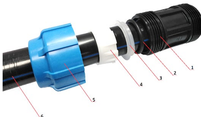
Рисунок 1- Конструкция компрессионной части фитинга.
