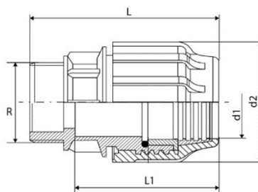
Рисунок 5 - Муфта с наружной резьбой
