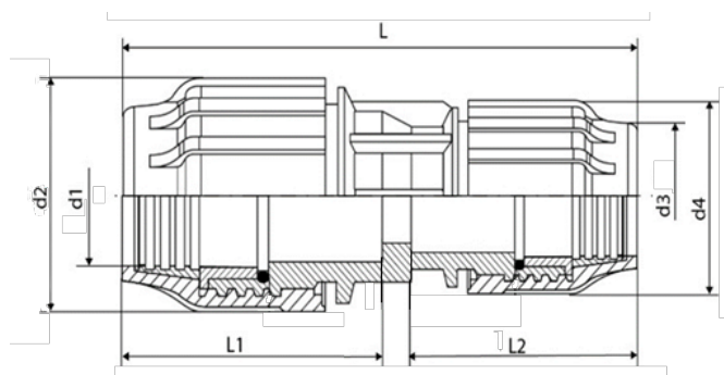
Рисунок 3 - Муфта переходная
