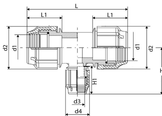
Рисунок 7 - Тройник переходной
