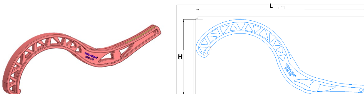
Рисунок 20 Ключ для гаек компрессионных фитингов dn 90-110 ТПК-АКВА
