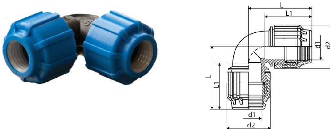
Рисунок 10 - Отвод 90°
